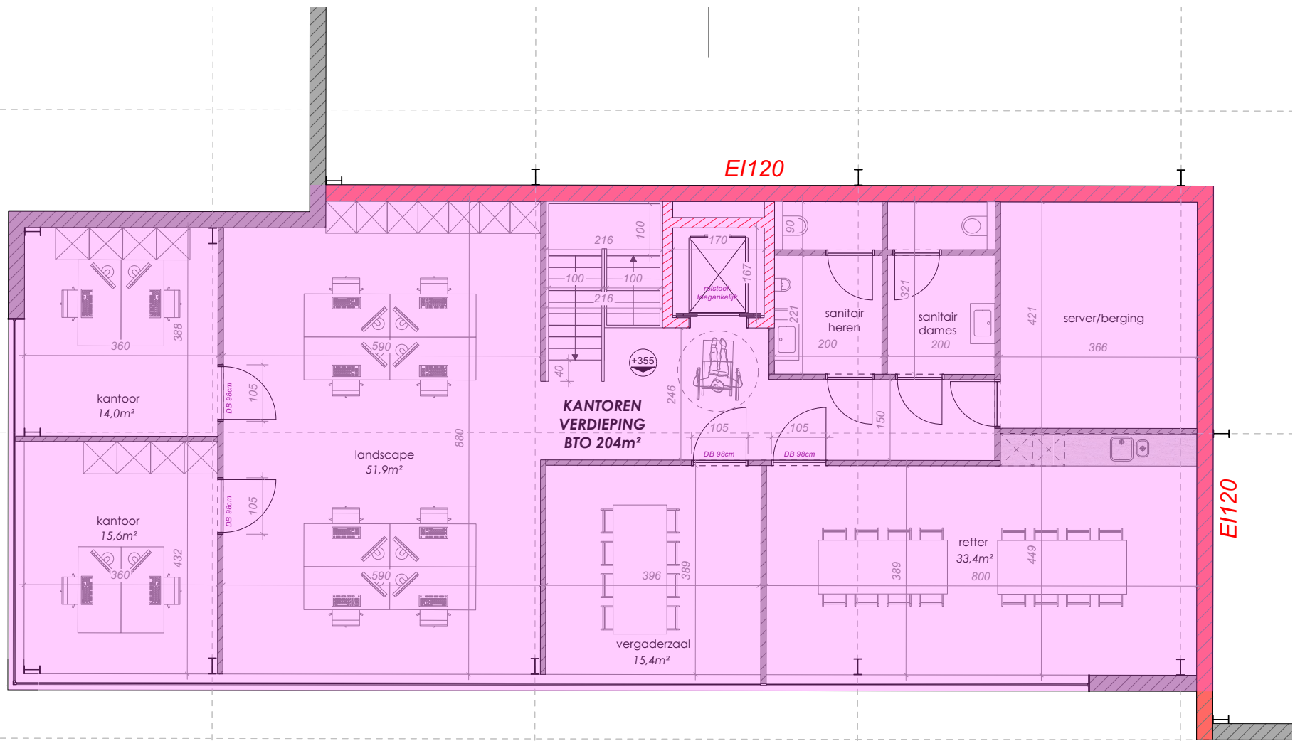
VERDIEPING
