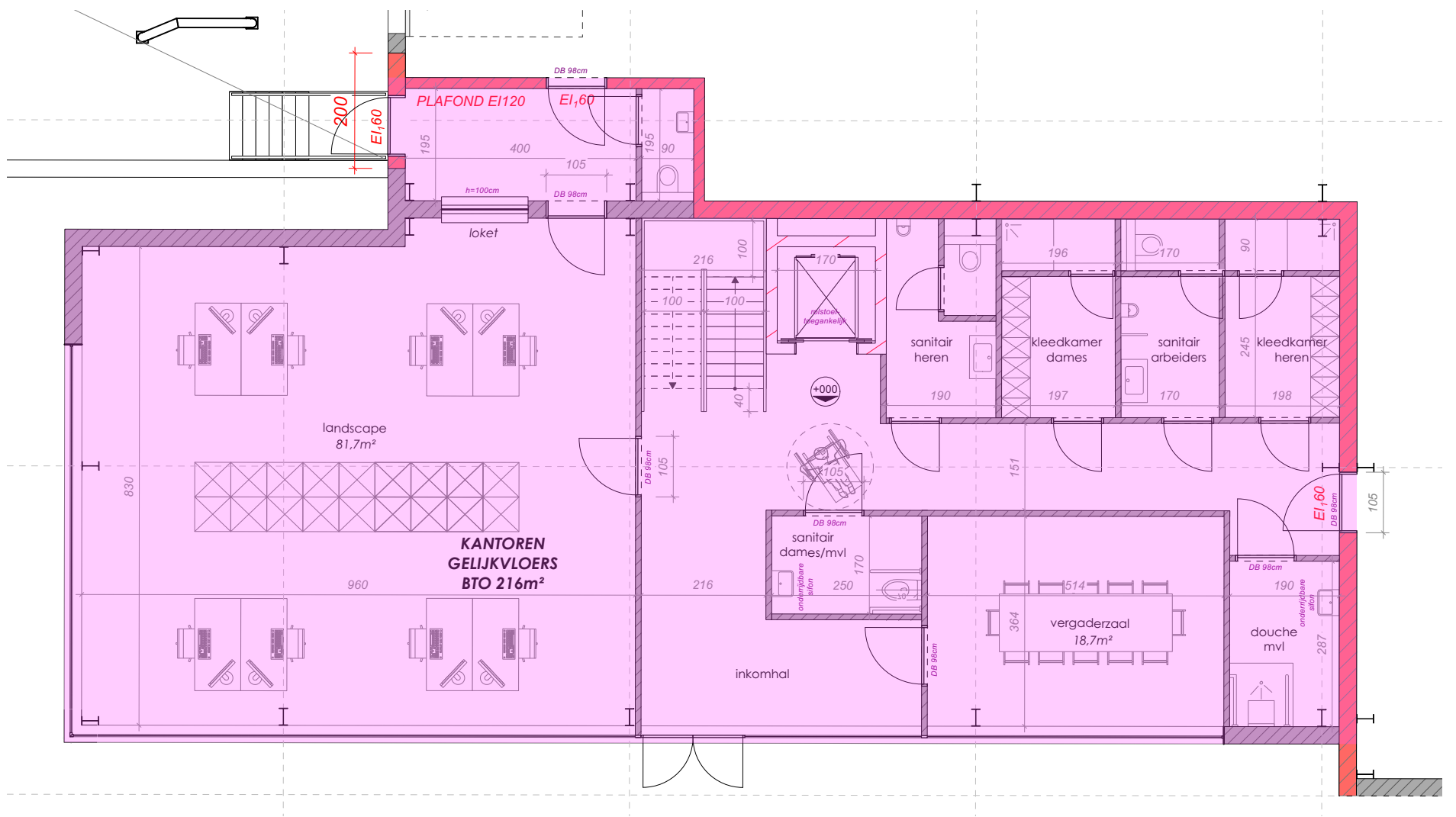
GRONDPLAN
